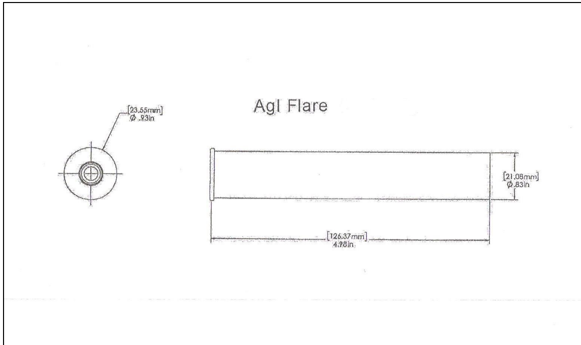
Διάγραμμα-1: Διαστάσεις φυσιγγίου Ιωδιούχου Αργύρου
